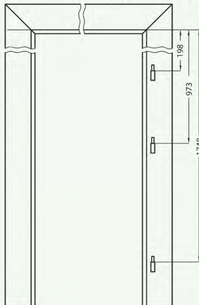
Vodorovný prierez
